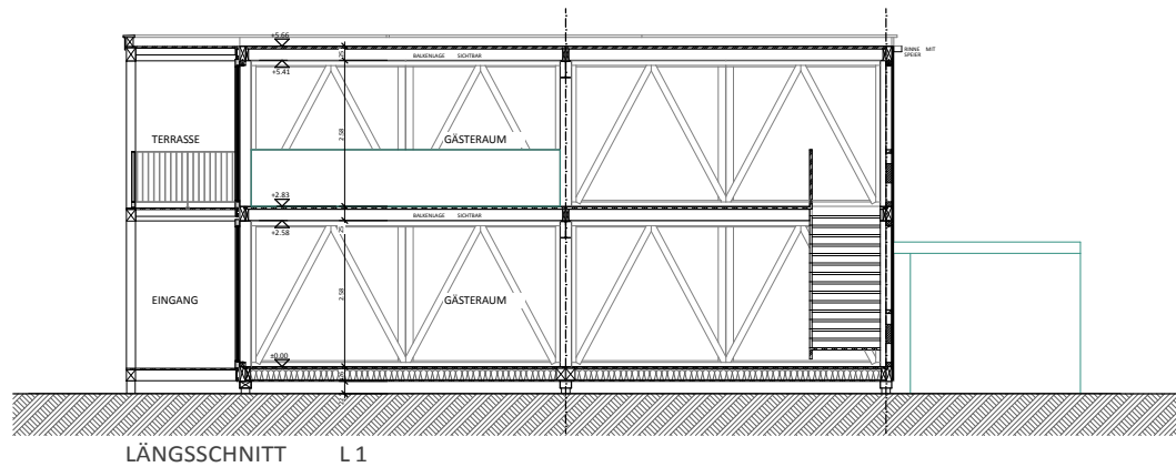
LÄNGSSCHNITT L 1
