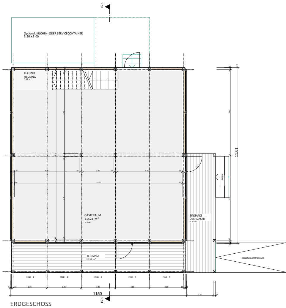
ERDGESCHOSS
